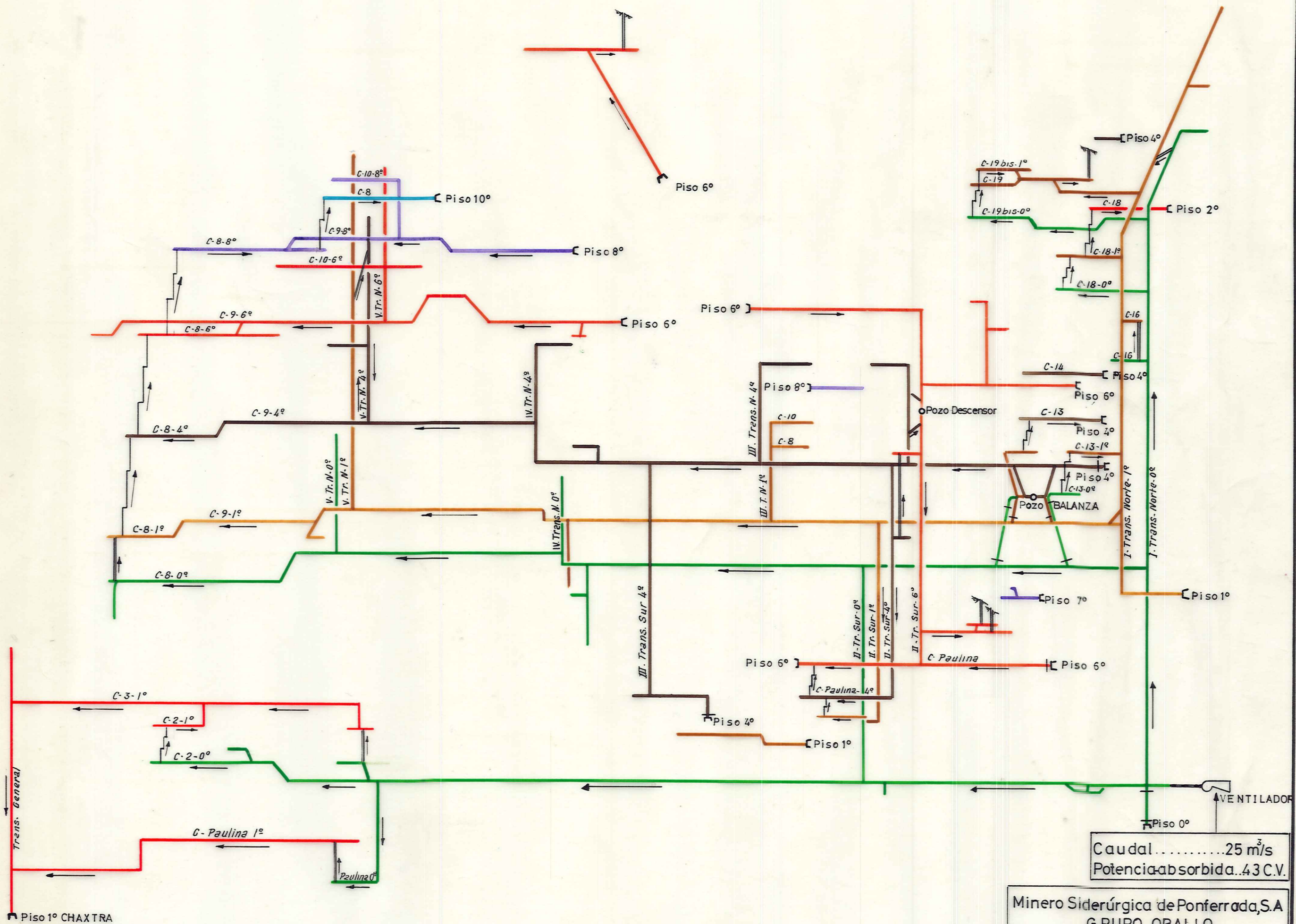
ESQUEMA DEL Circuito de Ventilación
