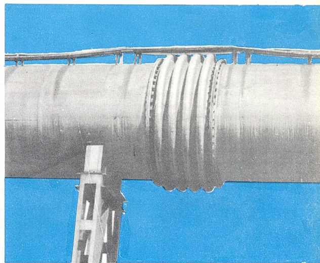
Fig. 4. - Compensación de dilatación de tuberías por medio de compensadores.
