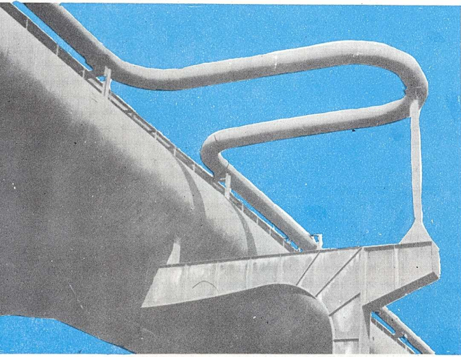
Fig. 3. - Compensación de dilatación de tuberías por medio de tiras.
